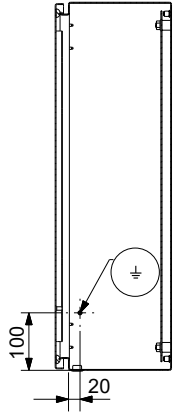
3-fach - mit Montageplatte / with Mounting plate 640x640x200mm Bestellnummer / Order Number: 400.17641 OHNE Ausschnitt / WITHOUT cutout
